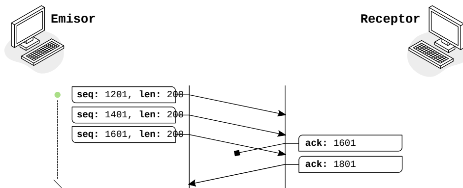
FIGURA 13.10: TCP: Confirmación perdida
