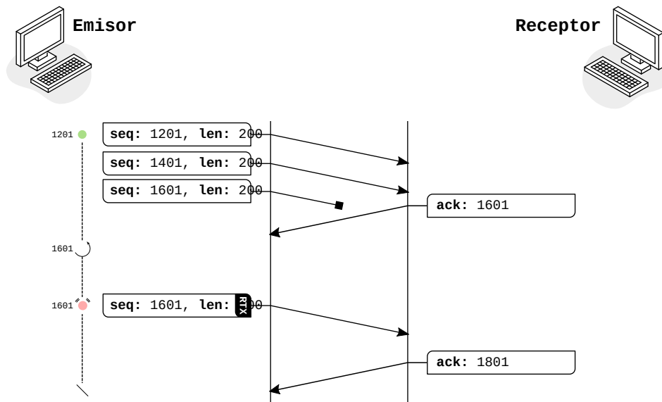
FIGURA 13.9: TCP: Segmento perdido
